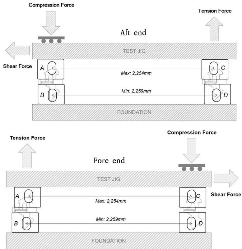
그림 3.25.2 HHS 시험장치 구성 (fully automatic twistlock) (2024)
