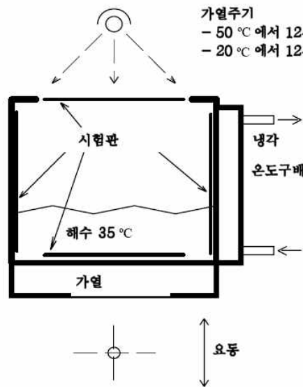
그림 3.30.2 밸러스트탱크 보호도장시스템의 시험을 위한 모의탱크
