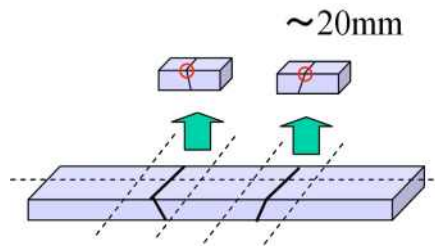
그림 3.32.8 시험편의 준비
