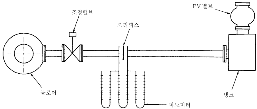
그림 3.24.1 PV 밸브의 시험장치
