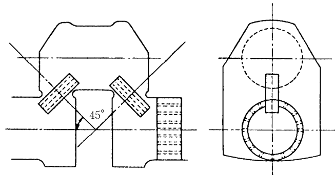
그림 2.5.3 굽힘피로시험편 채취위치
