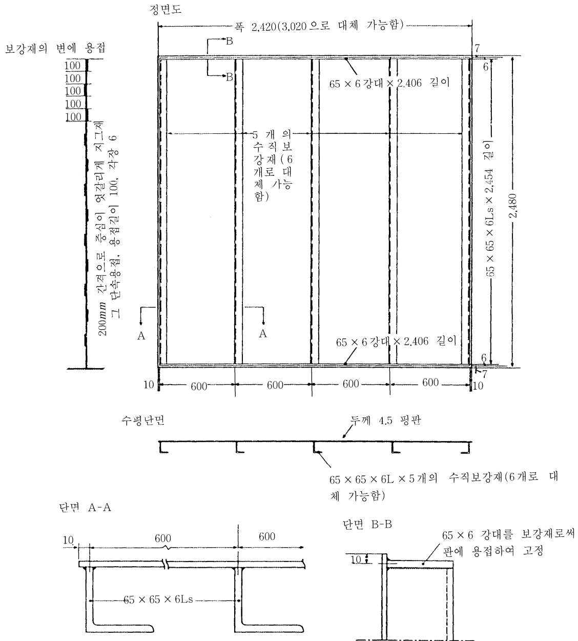
그림 3.26.2 A급 격벽 및 B급 내장재의 주요구조부재의 치수
