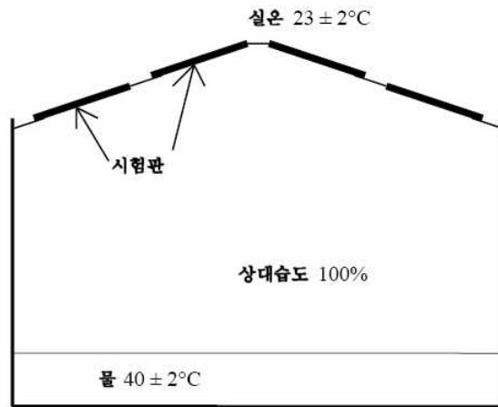
그림 3.30.3 응축체임버
